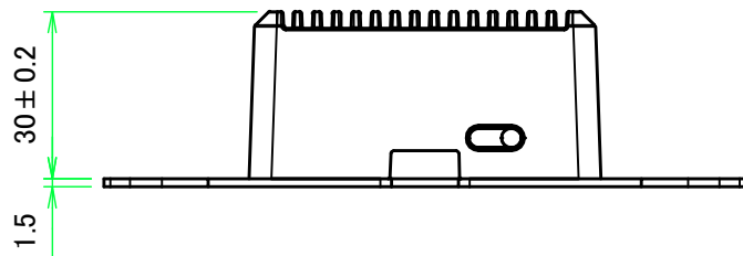
A-A ( 1 : 1.5 )
