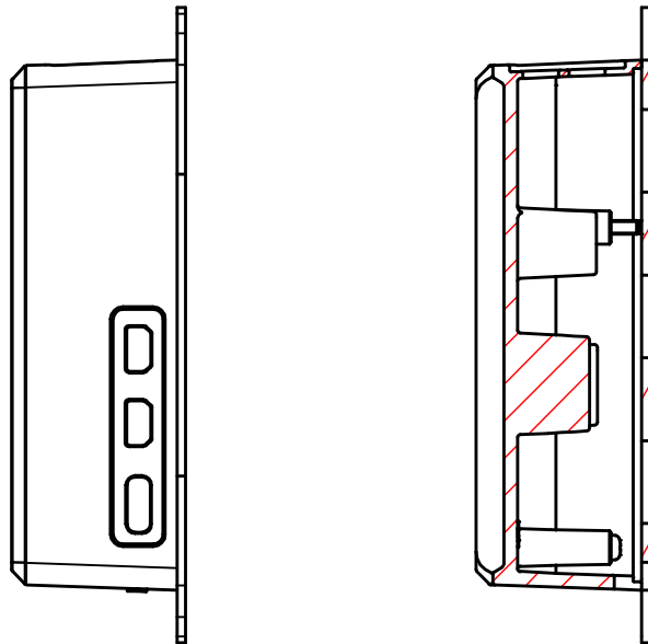
B-B ( 1 : 1.5 )
